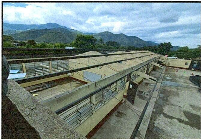
Foto 1: INSTALACION DE LÁMINA TROQUELADA EN AULAS Y DIRECCION. (MODULO I)
