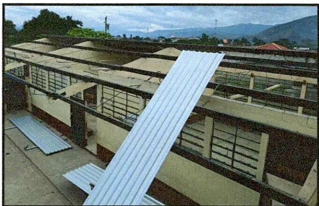
Foto 3: INSTALACION DE LÁMINA TROQUELADA EN AULAS. (MODULO II)
